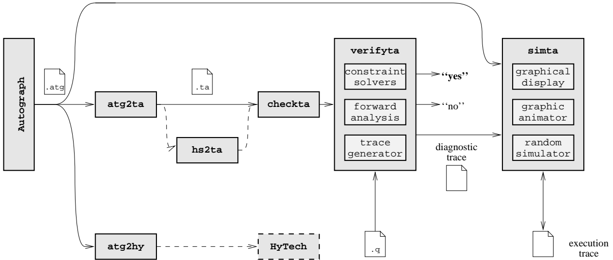
Fig. 1. Overview of UPPAAL
